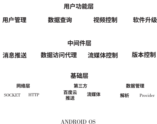
图2 智慧竞赛 APP 分层设计
